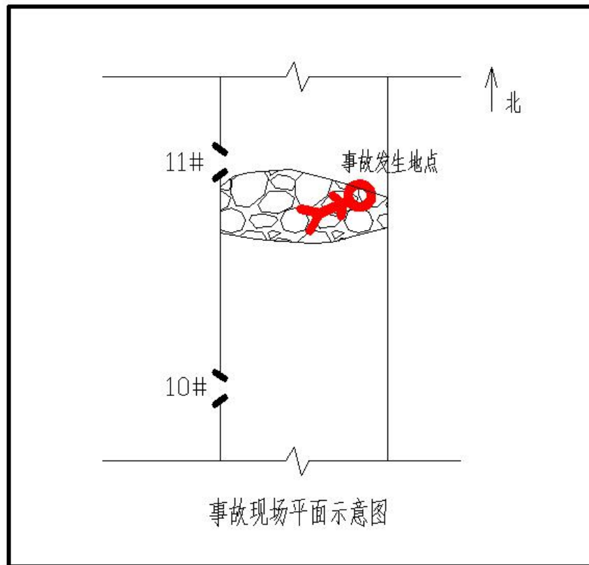
图四：事故现场平面示意图
