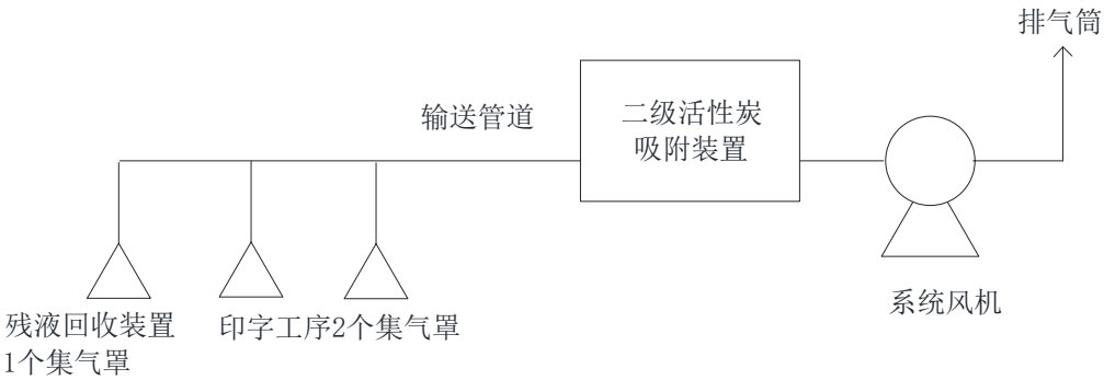
图 4-3 印字工序、残液回收装置泄漏废气治理系统集输管线图
