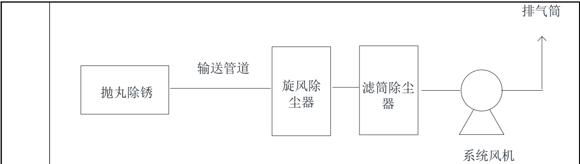
图 4-2 抛丸除锈工序废气治理系统集输管线图
