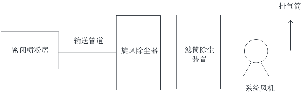
图 4-4 静电喷粉工序废气治理系统集输管线图
