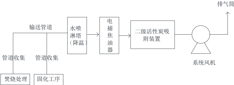
图 4-1 焚烧处理工序和固化工序废气治理系统集输管线图
