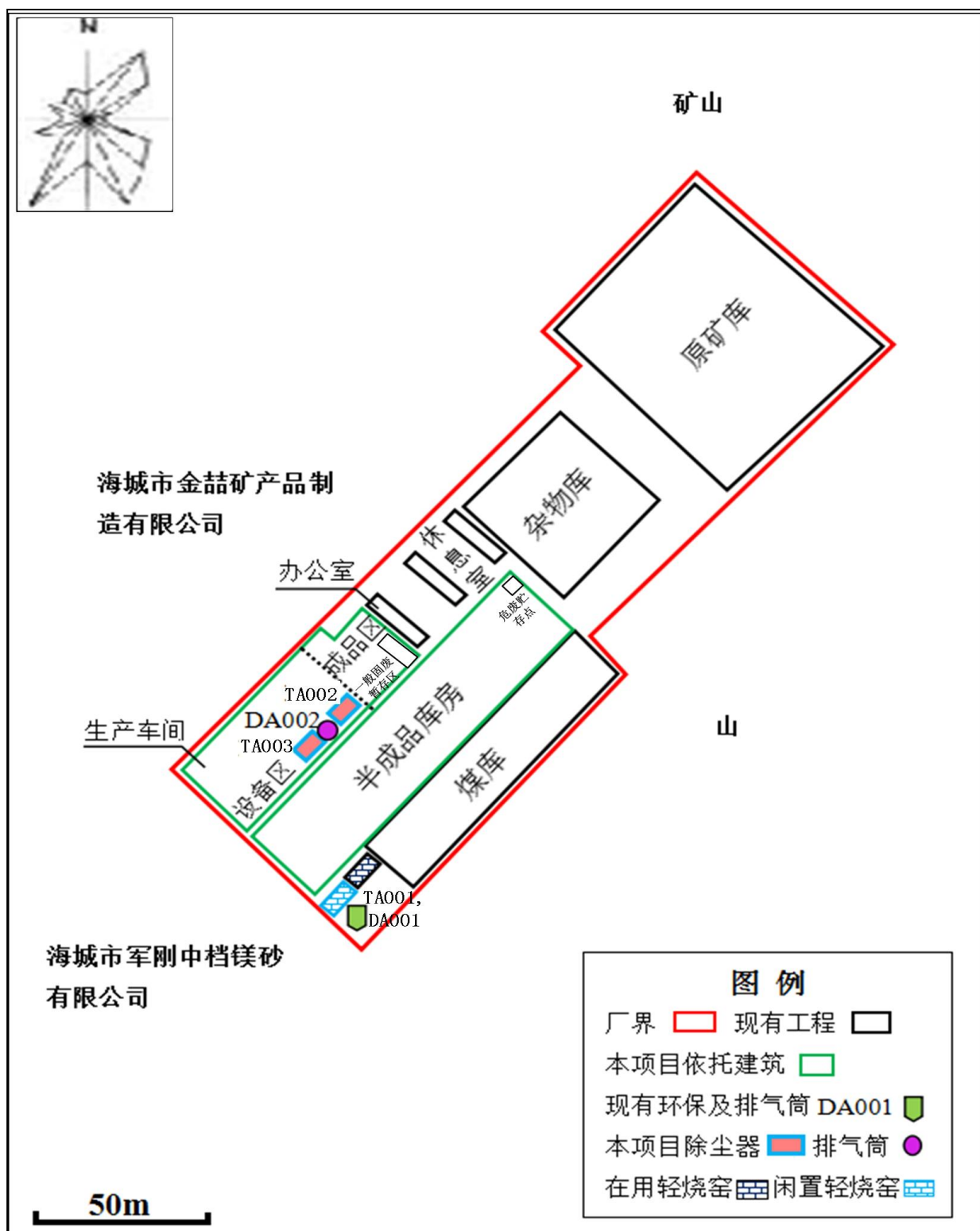
附图 2 全厂平面布置图
