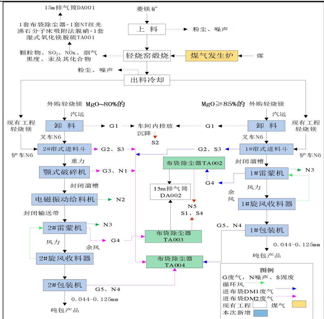
图 2-1 项目生产工艺流程及排污节点图
