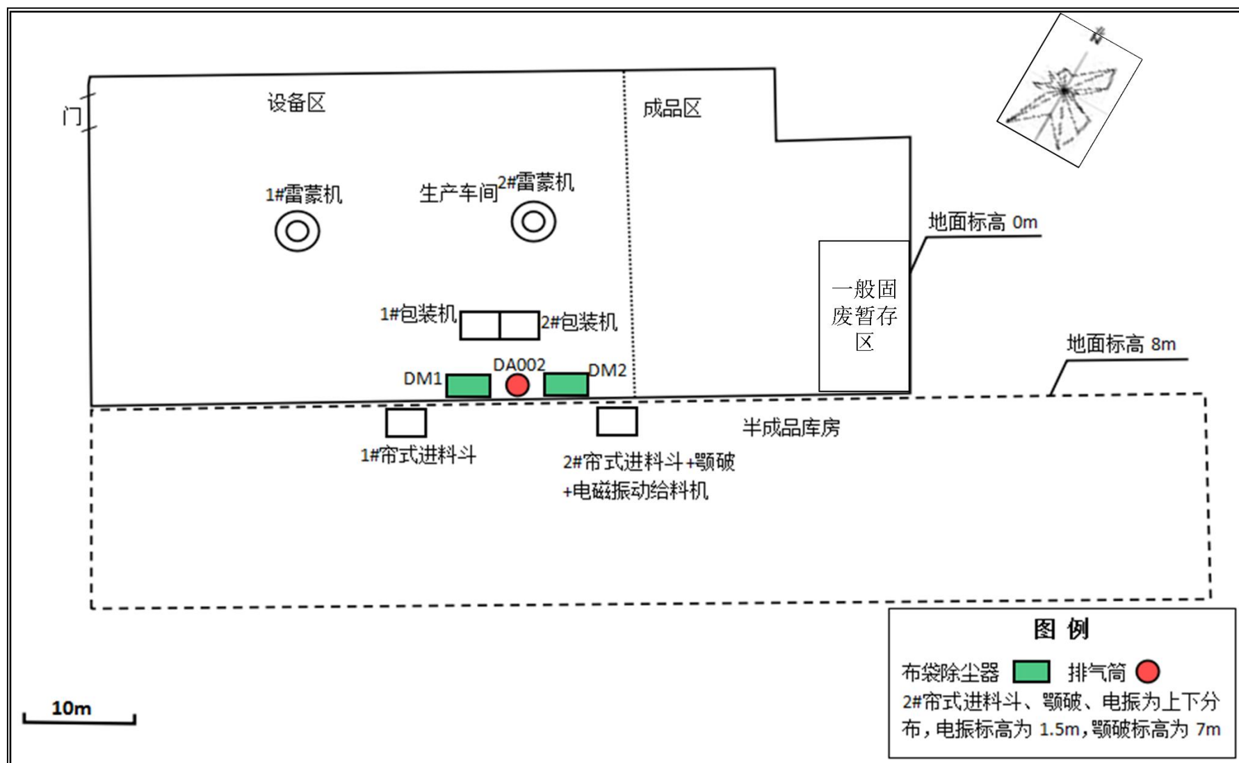
附图3 车间设备布局图（半成品库房仅示意封闭库）
