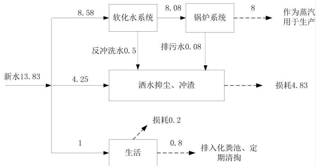
图 2 全厂水平衡图 (t/d)
