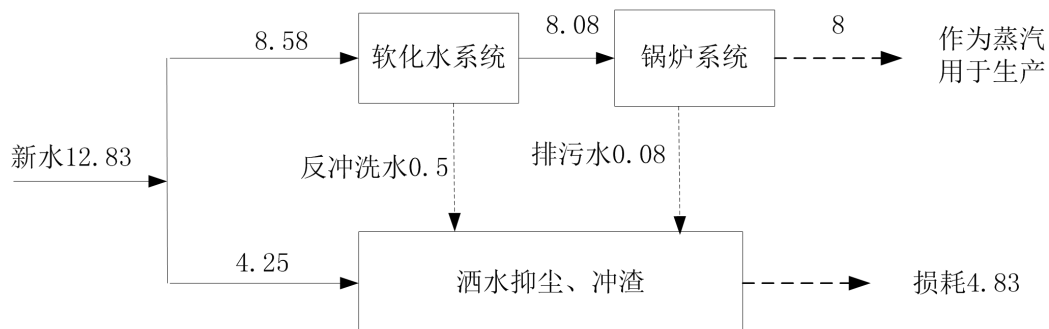
图 1 本项目水平衡图 (t/d)
