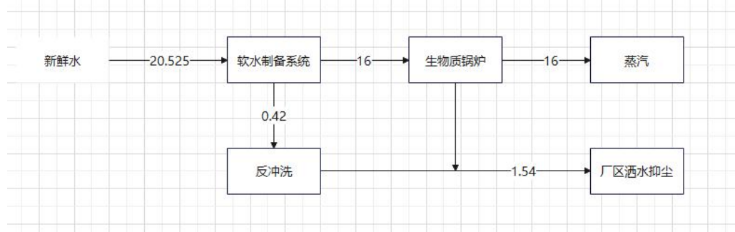
图 2-1 水平衡图 (m³/d)
