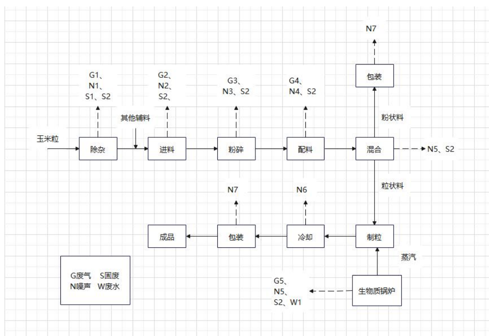
图 2-2 工艺流程及产污节点图
