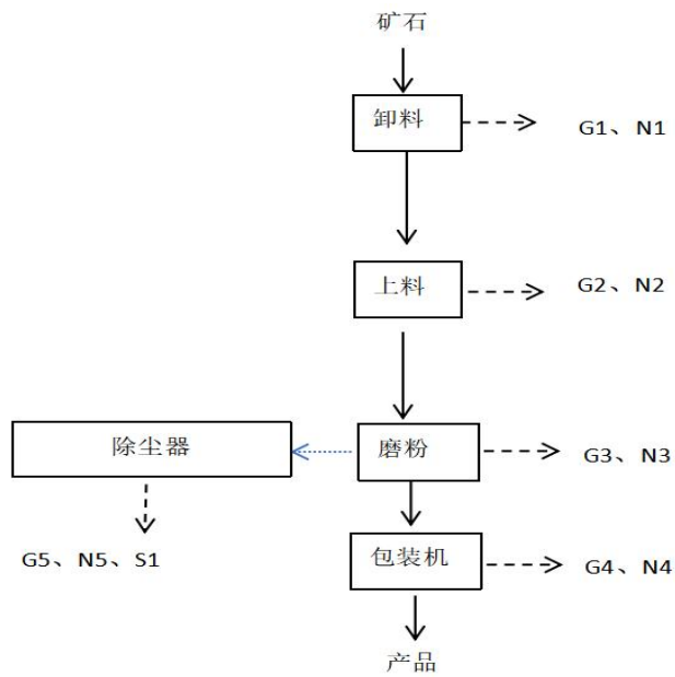
图 2-1 工艺流程及排污节点图（废气 G、噪声 N、固废 S）
