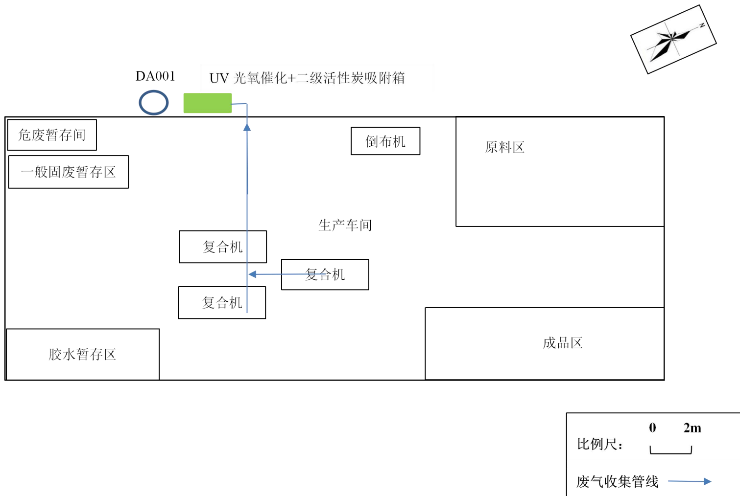
附图 4 (b) 拟建项目车间平面布置图
